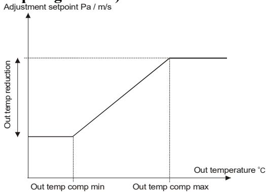
Figuur 2: Buitentemperatuur compensatie.
